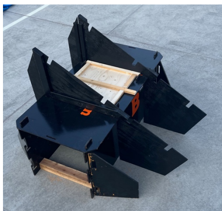
④ サイドパネルを差し込む
